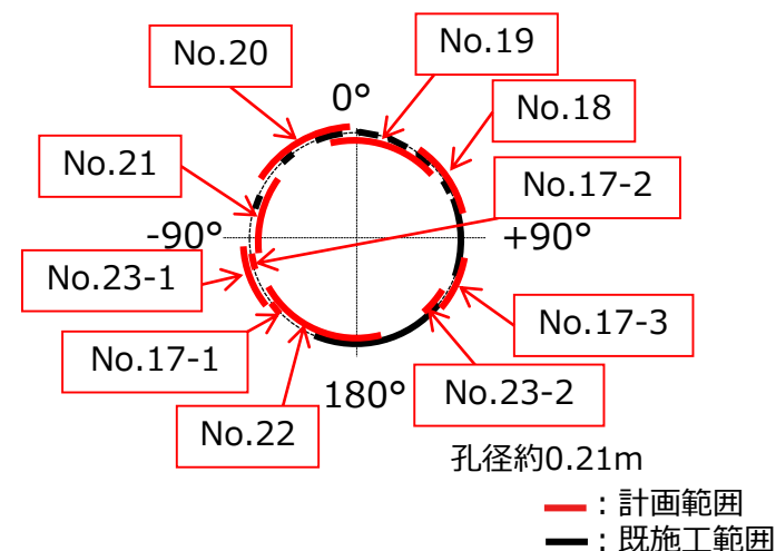
切削範囲イメージ (紙面奥側がPCV内側)
